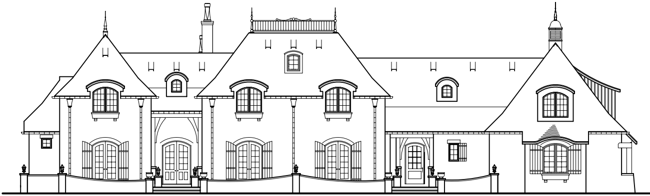
E1 FRONT ELEVATION
