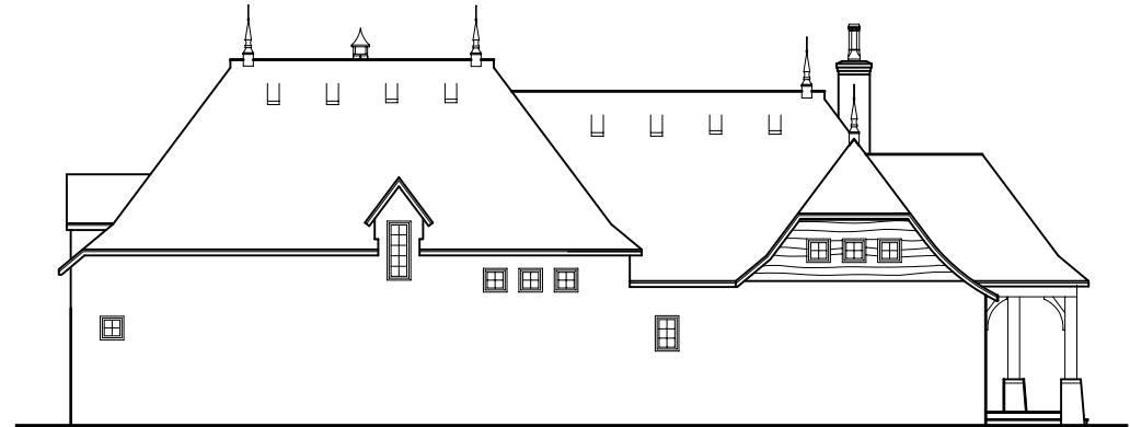
E4 RIGHT ELEVATION
